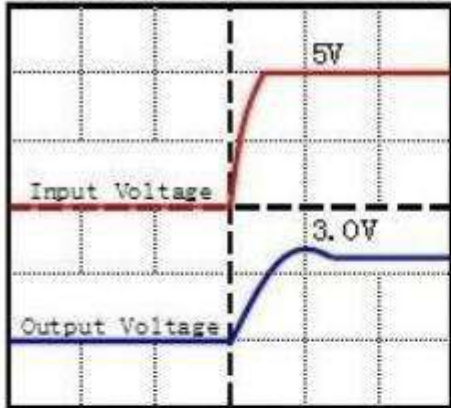
CY7330-ATR Iout=10mA CL=10uF
