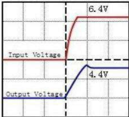
CY7344-ATR Iout=10mA CL=10uF
