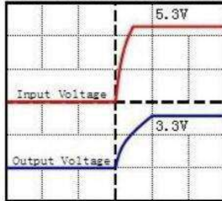
CY7333-ATR Iout=10mA CL=10uF
