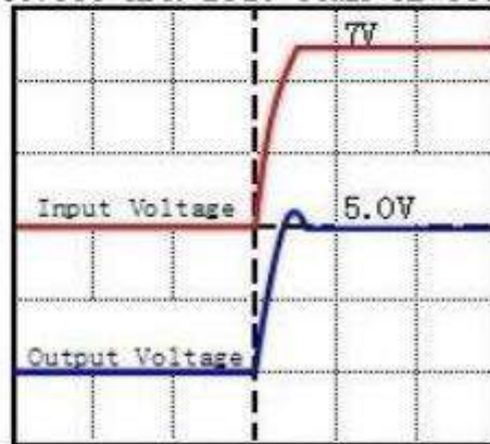
CY7350-APR Iout=10mA CL=10uF
